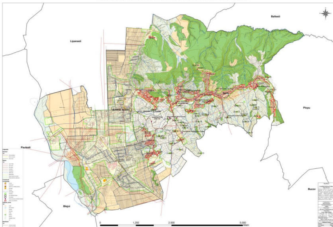
Harta zonelor de risc la alunecari de teren a Orasului Boldesti - Scaieni
