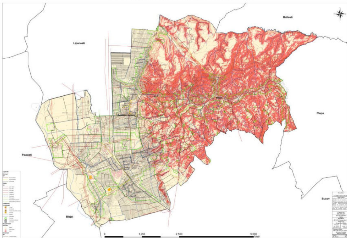
Harta de hazard la alunecari de teren a Orasului Boldesti-Scaieni
